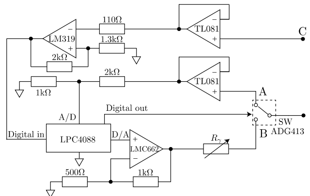
疑似生成した周期振動を安定化する制御器のプロトタイプ
