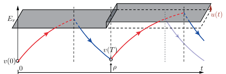
しきい値振動型システム安定化制御法のイメージ図
