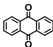
アントラキノン
