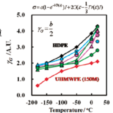
Fig.1 低温特性と非調和性との相関
