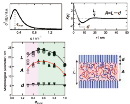
結晶性/非晶性高分子の結晶ラメラ構造の解析
