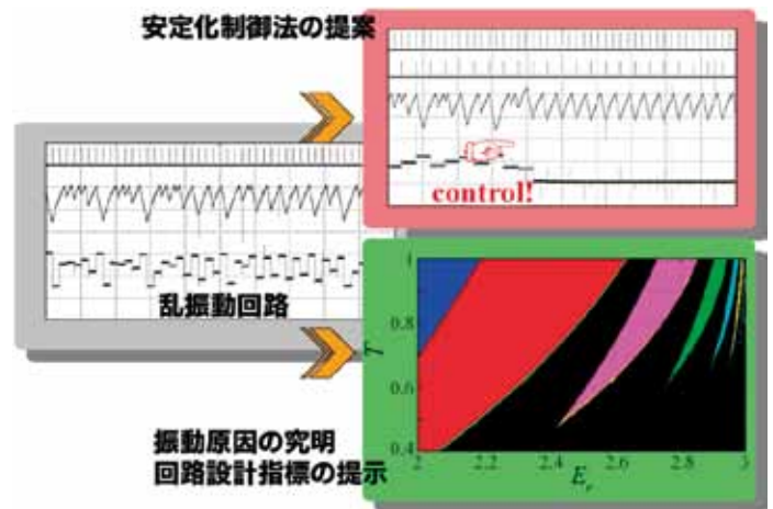
乱振動回路の安定化制御と回路解析
