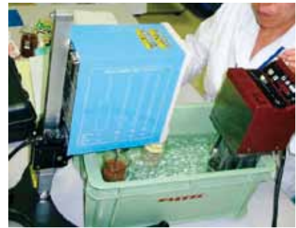
B型粘度計による 粘度の測定
