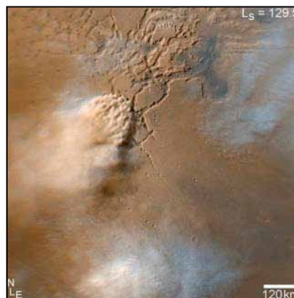
↑ Mars Reconnaissance Orbiter搭載のMars Color Imagerによって撮影された火星のダストストーム。
