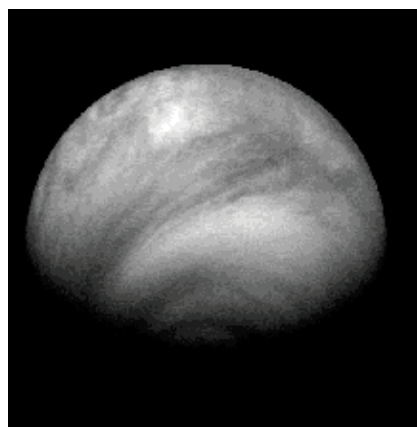
↑ Venus Express搭載のVenus Monitoring Cameraによって撮影された金星の紫外画像。
