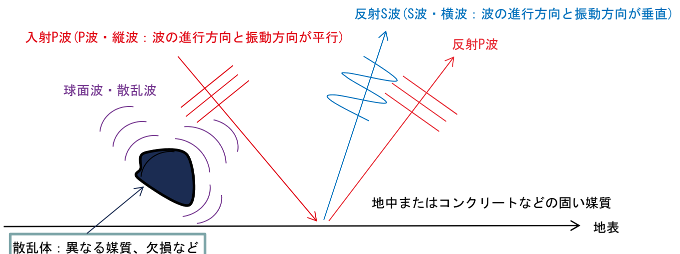
半無限領域で散乱体を仮定した弾性波の伝播のイメージ
