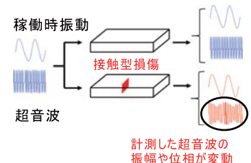
図3 損傷による非線形振動現象
