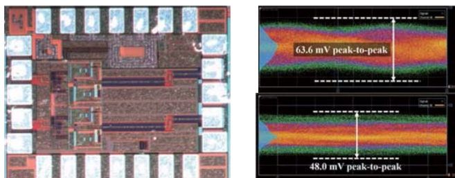
(a) チップ写真 (b) ノイズ波形(上: 従来/下: 提案)
